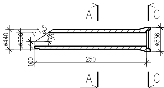
PRZEKRÓJ B-B
