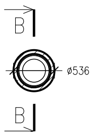
PRZEKRÓJ C-C
